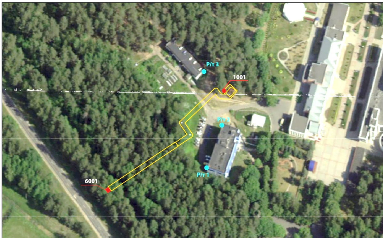
Рисунок 4.1 – Расположение расчетных точек (Р/т) на границе жилой зоны
